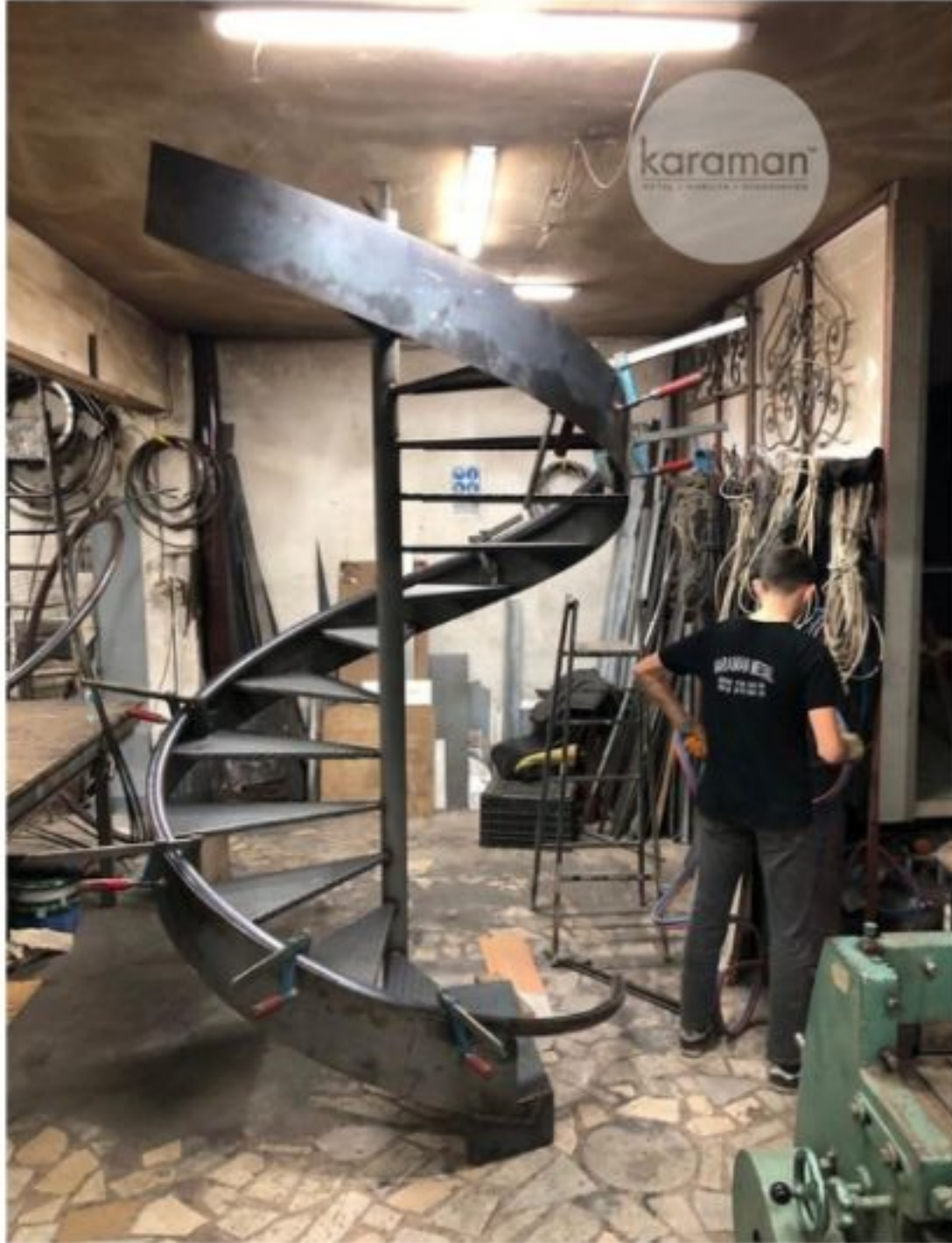
Çelik Konstrüksiyon, Fırın Boyalı Döner Merdiven Çalışmamız •HGOOffice,Ataşehir • İstanbul
