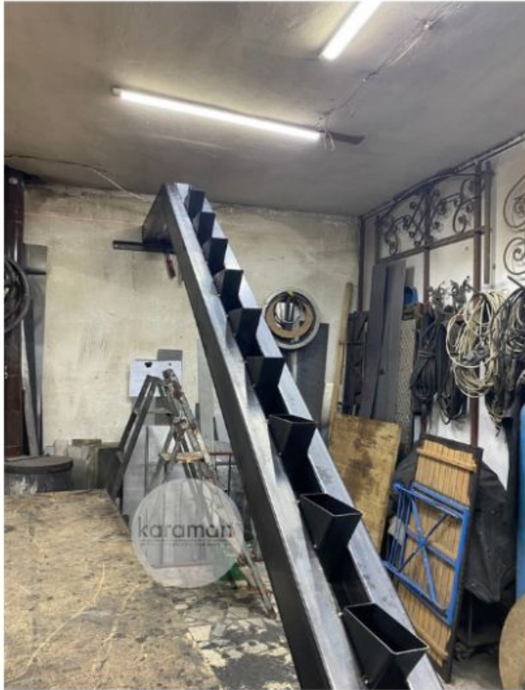
Çelik Konstrüksiyon, Fırın Boyalı, Tek Omurga Sistemli Merdiven Çalışmamız •C.K.Evi,Amsterdam • Hollanda
